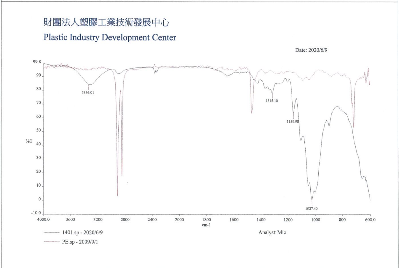
附圖二：紅外線光譜分析圖(樣品與PE疊圖)
