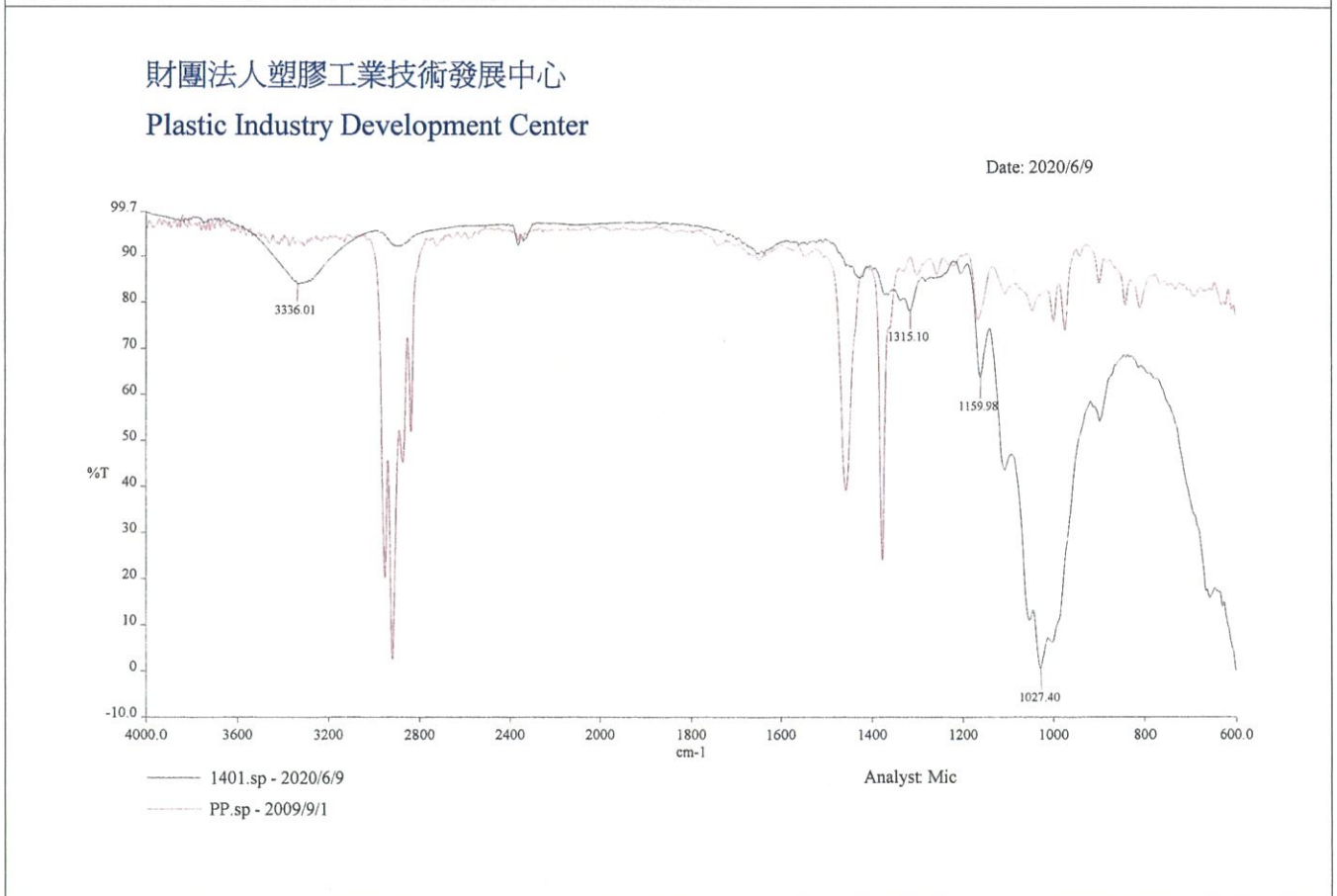
附圖一：紅外線光譜分析圖(樣品與PP疊圖)
