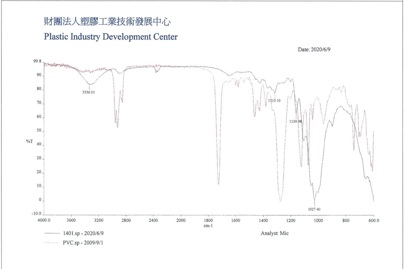
附圖四：紅外線光譜分析圖(樣品與PVC疊圖)
