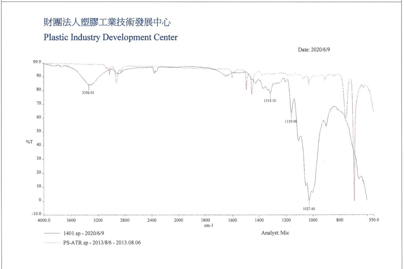
附圖三：紅外線光譜分析圖(樣品與PS疊圖)
